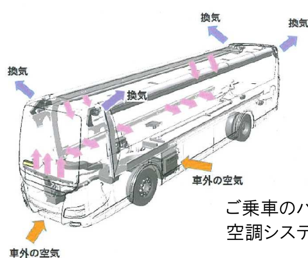
大型観光バス・床下A/Cタイプ
