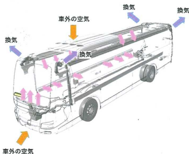
大型観光バス・天井A/Cタイプ
